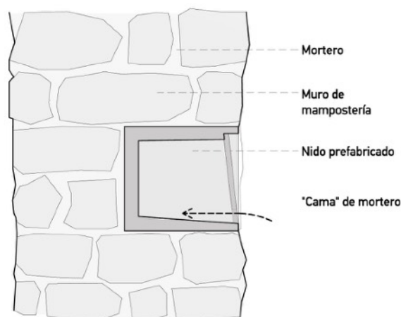
SECCIÓN
